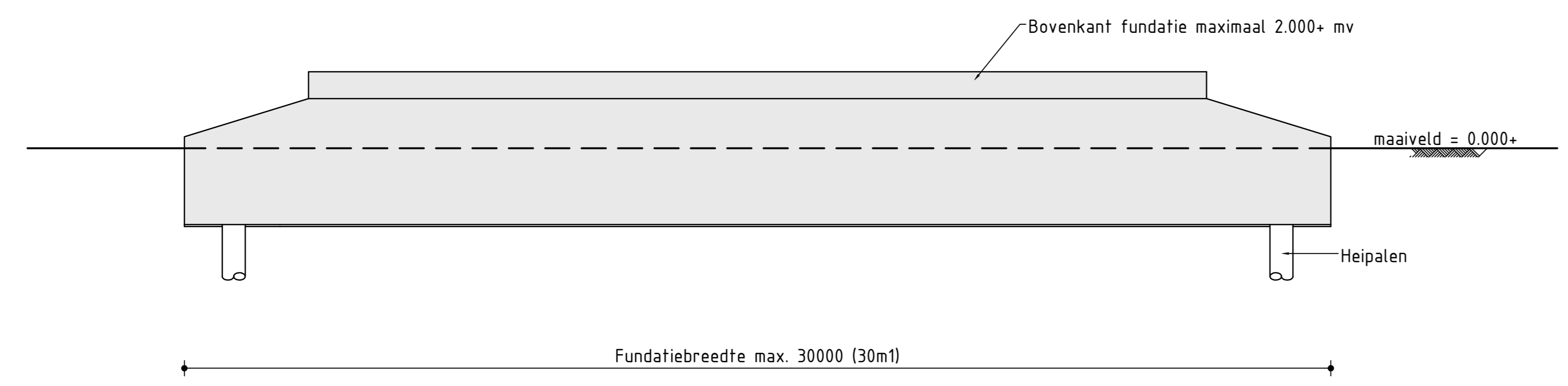
Principe Detail paalfundatie Schaal 1 : 100
