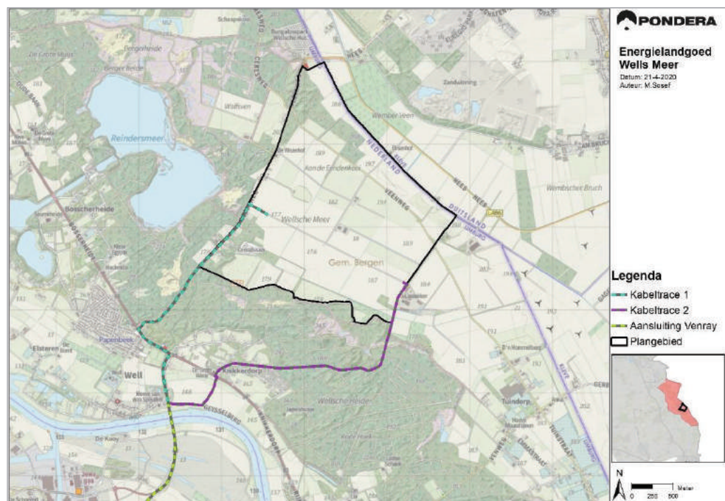
Figuur 1.5 Kabeltracés
