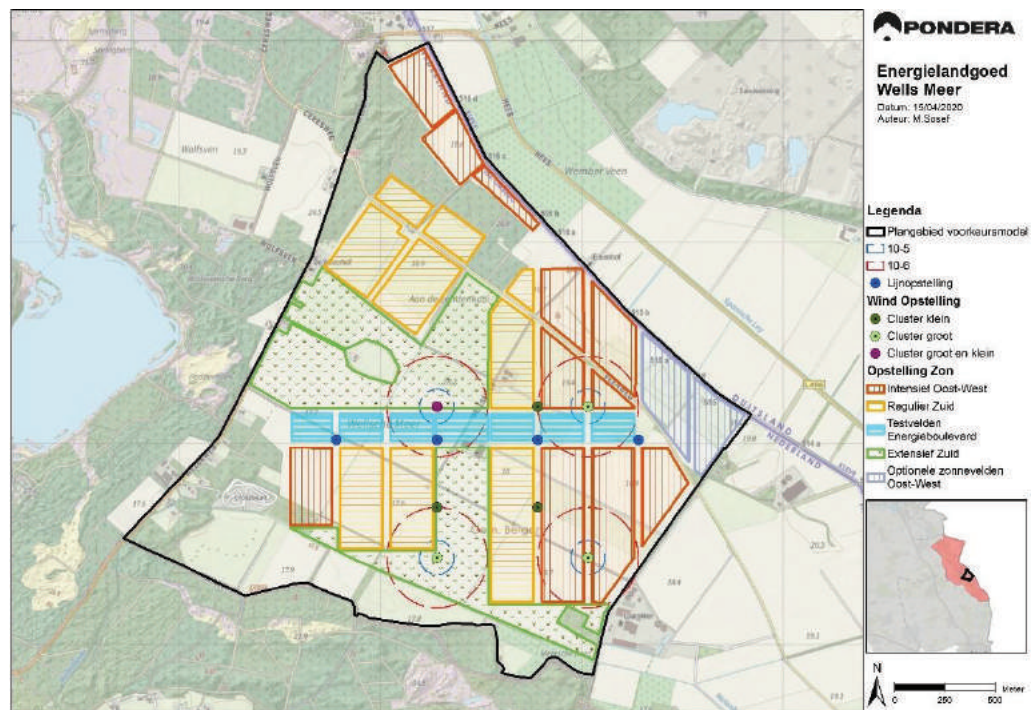
Figuur 17.38 Risicocontouren windturbines VKM 2B - clusteropstelling groot
