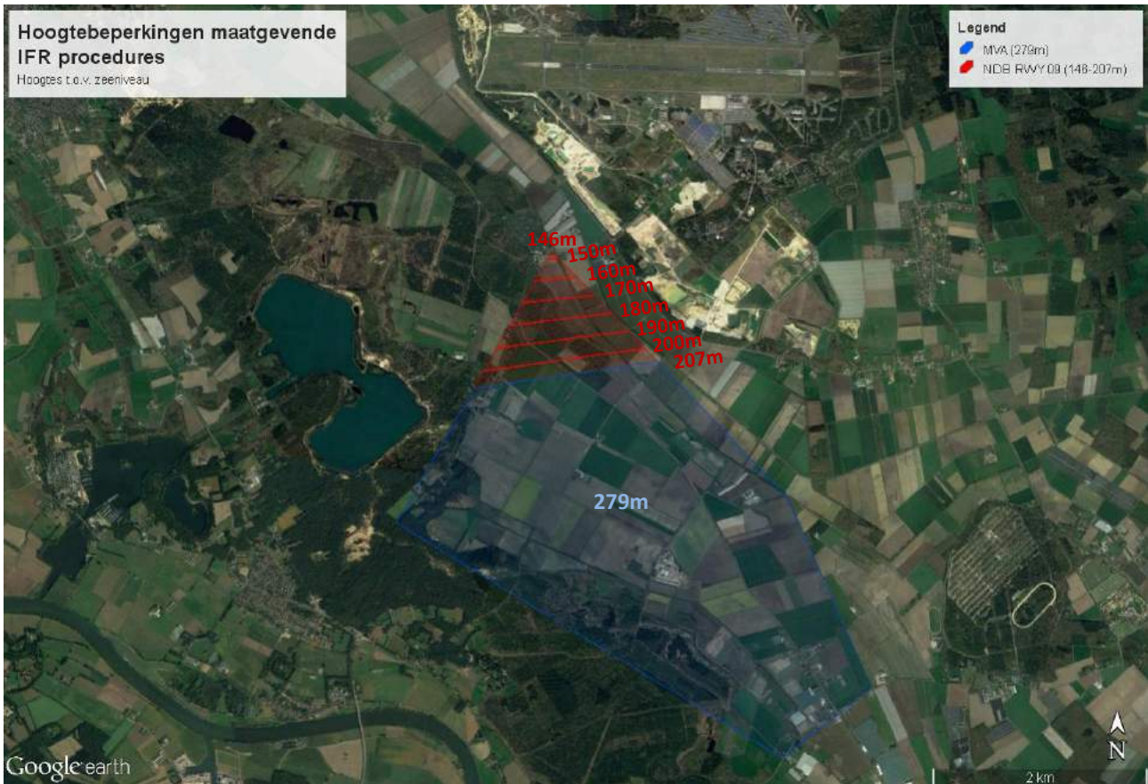
Figuur 3-3: Hoogtebeperkingen voor plangebied Wells Meer als gevolg van de maatgevende instrumentvlieprocedures van luchthaven Weeze
