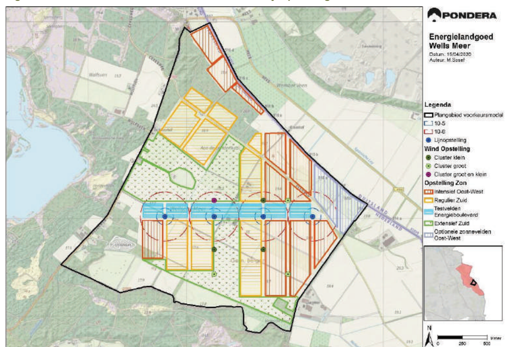
Figuur 17.36 Risicocontouren windturbines VKM 1 – lijnopstelling
