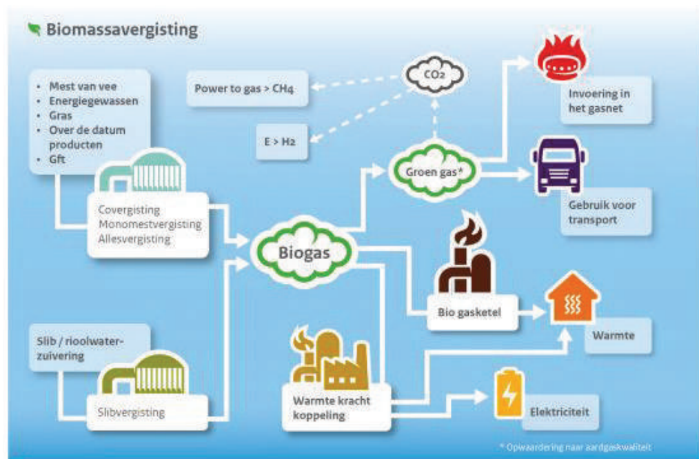
Figuur 4.2 schematische weergave biomassa vergisting.
