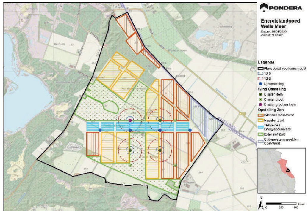
Figuur 17.37 Risicocontouren windturbines VKM 2A - clusteropstelling klein
