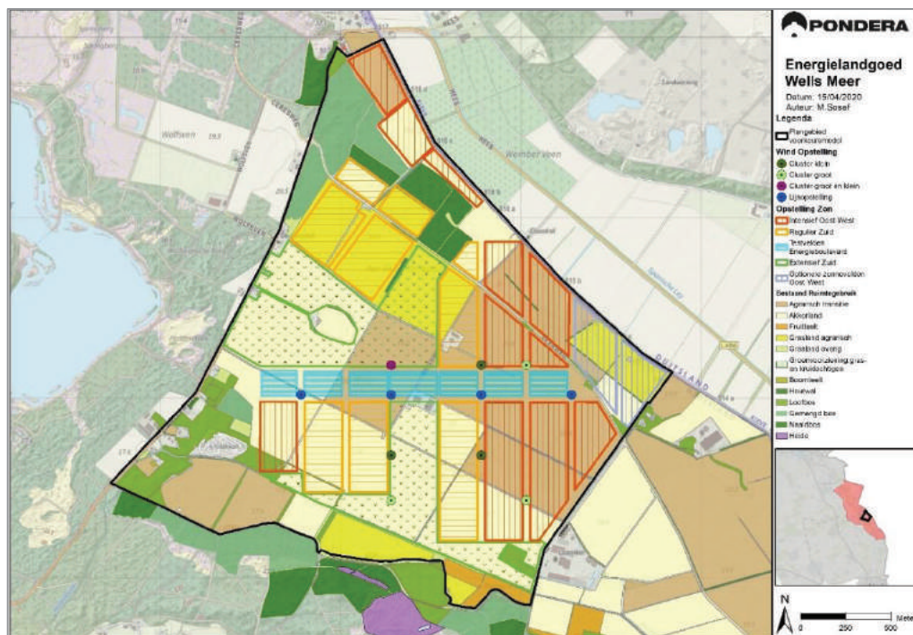
Figuur 17.34 Wind- en zonne-energie opstellingen in het voorkeursmodel
