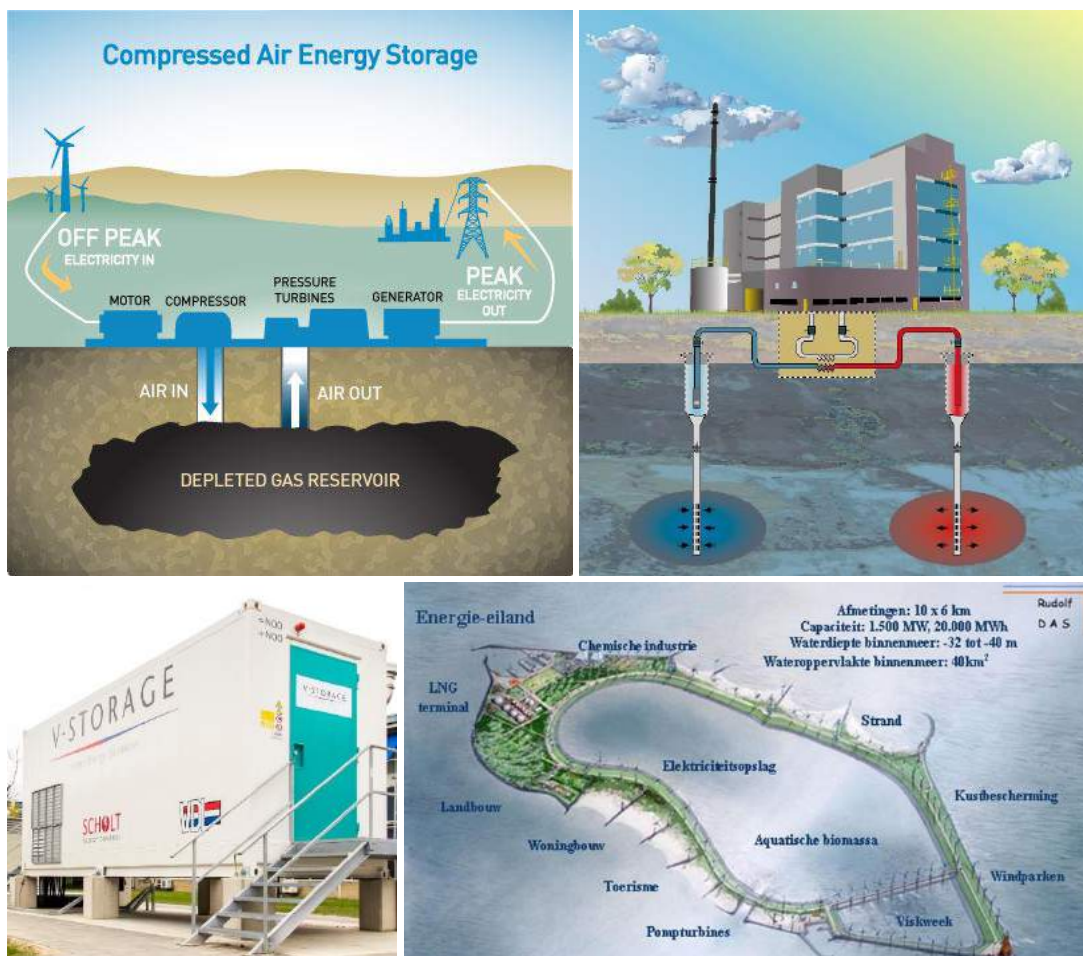
Figuur 6.5: Compilatie van verschillende vormen van energieopslag. Met de klok mee: samengeperste lucht, een WKO-systeem, het Energie-eiland met o.a. pompaccumulatie en een V-storage batterij. (Bron: diversen online)
