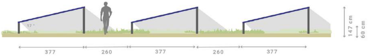
Doorsnede zonnepanelen met indicatie van de maatvoering. Deze opstelling gaat uit van vier panelen boven elkaar, landscape.
